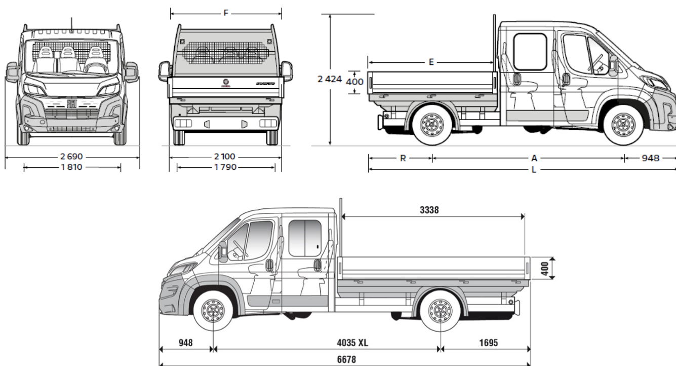
Габаритні розміри та розміри вантажного відділення, мм
