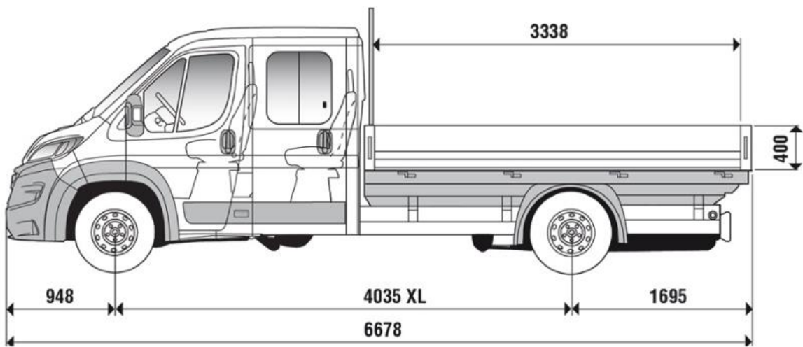
Габаритні розміри та розміри вантажного відділення, мм
